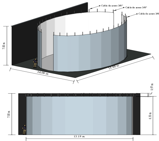
Plano 1. Plano del espacio escénico. Miradas laterales. Escala 1mm: 120 mm
