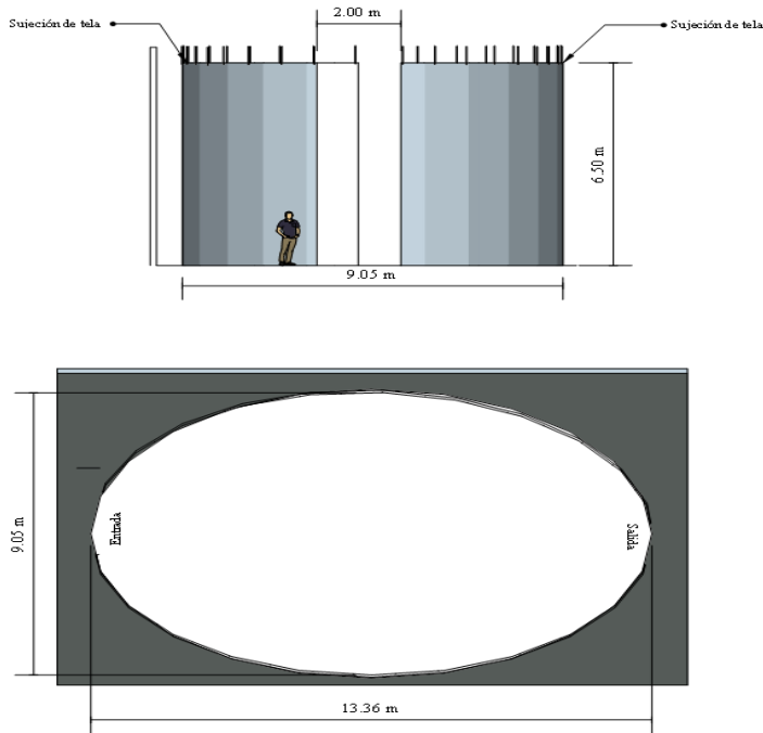
Plano 2. Plano del espacio escénico. Alto, ancho y largo. Escala 1mm: 120 mm
